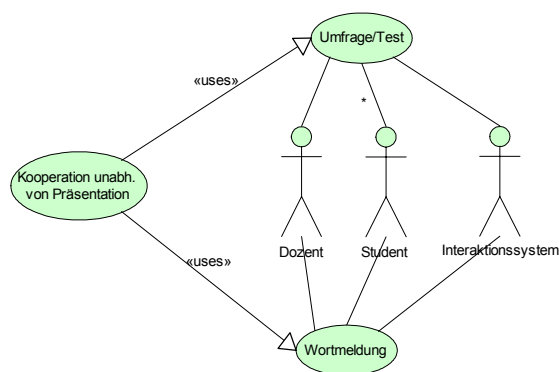
Abb. 1 Anwendungsfall Kooperation und abgeleitete Anwendungsfälle
