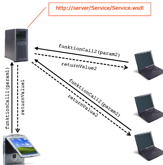
Abb. 3 Client/Server Architektur mit SOAP
