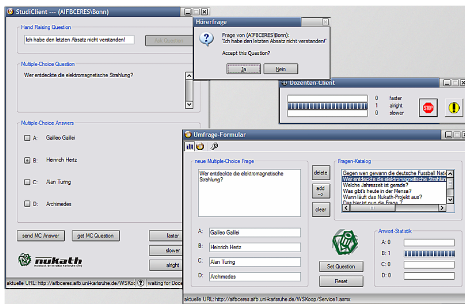
Abb. 2 Dozenten und Studenten Clients, Standalone-Versionen
