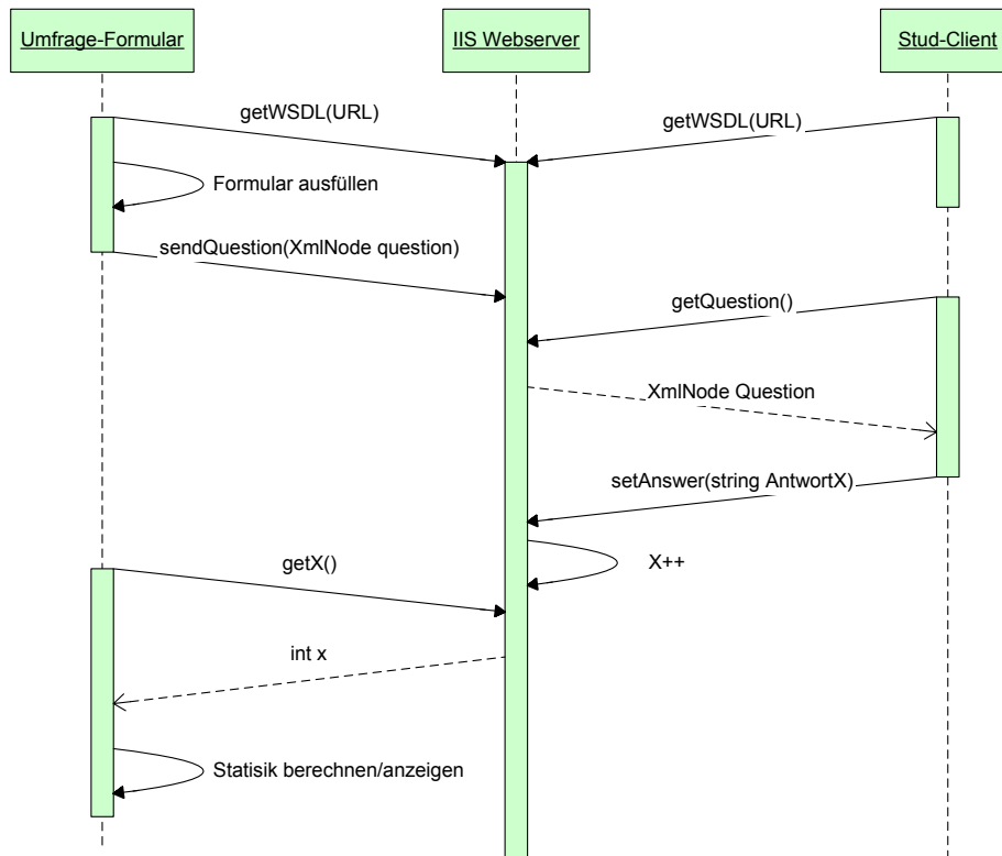
Abb. 4 UML-Sequenzdiagramm für das Multiple-Choice Szenario
