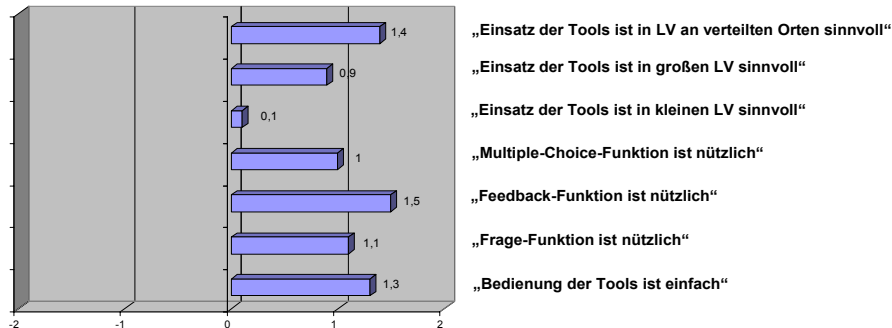
Abb. 5 Evaluationsergebnisse
